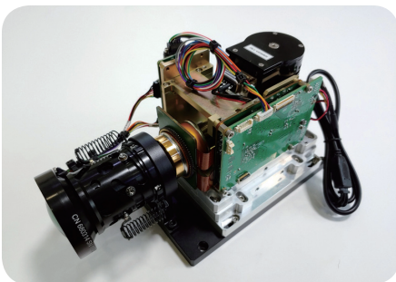
냉각식 열화상카메라 모듈 <SM-640>
